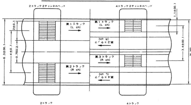
トラックの位置及び寸法（JISによる）
